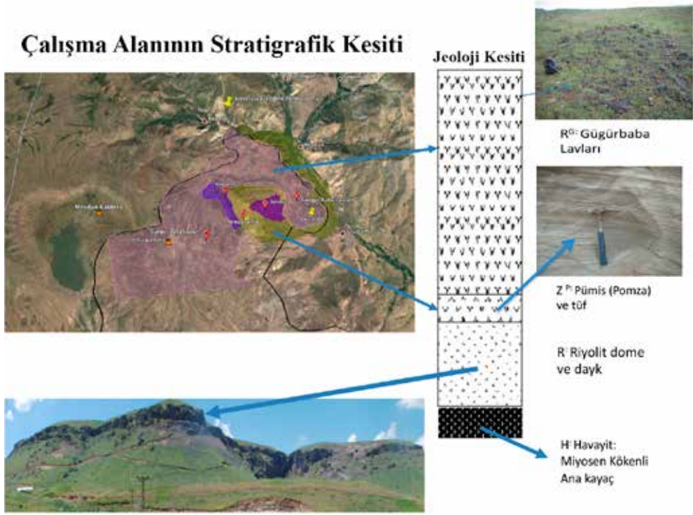
Figür 1: Gürgürbaba Tepesi jeolojik kesiti
