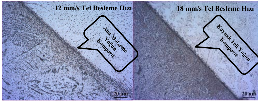
Şekil 8. Farklı tel besleme hızlarında mikroyapı görüntüleri
