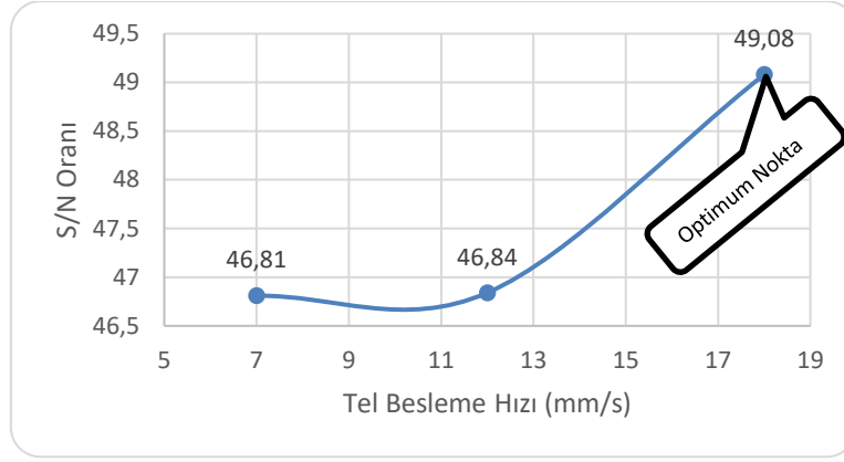
Şekil 7. Tel besleme hızı için hesaplanmış S/N oranları
