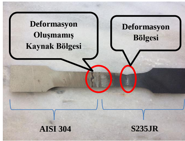
Şekil 4. S235JR bölgesinden deforme olmuş numune (enerji: 74,16 kJ, besleme hızı: 7 mm/s).
