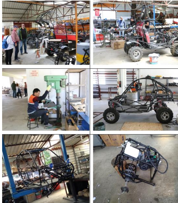
Fotoğraf 3. Buggy Cross Makinaları Üretim İstasyonu ve Çeşitli üretim aşamalarından görüntüler
