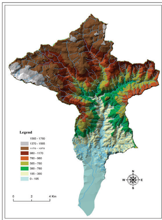
Fig.3. Elevation Level
