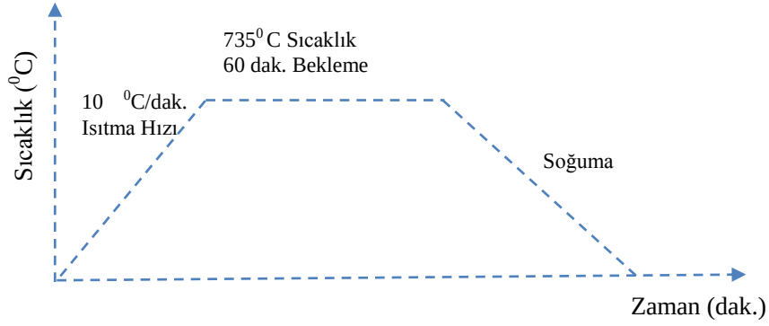
Şekil 3. Koruyucu Atmosferli Fırında Isıtma İşlem-Zaman Süreci
