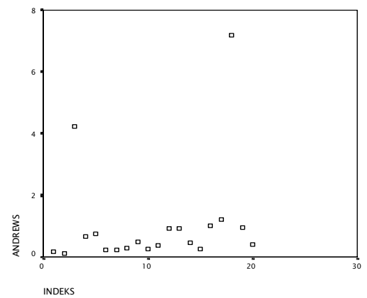
Şekil 5. ANDREWS Mutlak Hata İçin Indeks Plot
