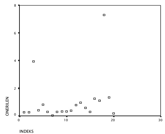
Şekil 6. ÖNERİLEN Mutlak Hata İçin Indeks Plot
