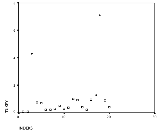
Şekil 4. TUKEY Mutlak Hata İçin Indeks Plot
