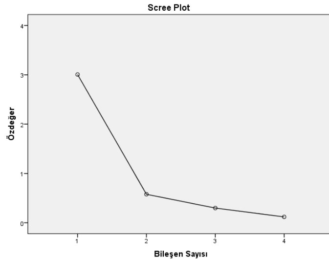
Şekil 1. Scree Plot Grafiği
