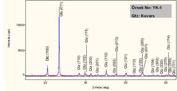
Şekil 20. Mavi-kahvemsıkızıl kalsedon + kuvars (Şekil 18-B) örneğindeki mikro kristalli kahvemsıkızıl kalsedon seviyelerinin XRD çekimi
