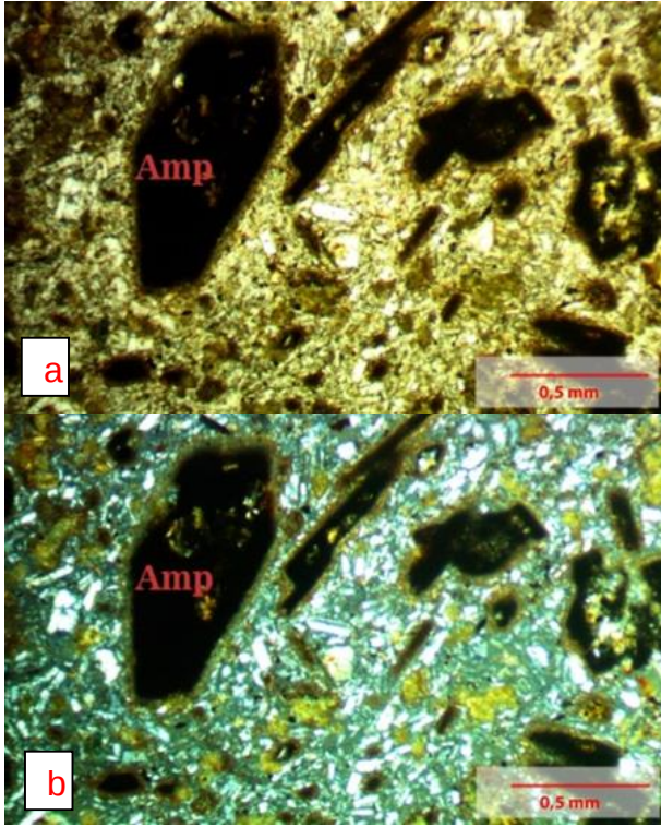
Şekil 11. Aydıncık batısı Keşlik mevkiinden alınan yan kayaç örneklerinde tamamıyla altere olmuş özşekilli amfiboller(kersutit) tek nikol (a), çift nikol (b).
