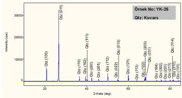
Şekil 23. Beyaz kalsedon+kuvars (Şekil 18-E) örneğindeki iri kristalli beyaz kuvars seviyelerinin XRD çekimi
