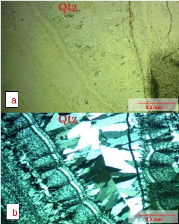
Şekil 16. Aydıncık batısı Keşlik mevkiinden alınan kalsedon örneğinde kenarlarda lifsi/iğnemsimikrokristalli ve merkezde makrokristalli kuvarsın tek nikol (a), çift nikol (b) görünümü.
