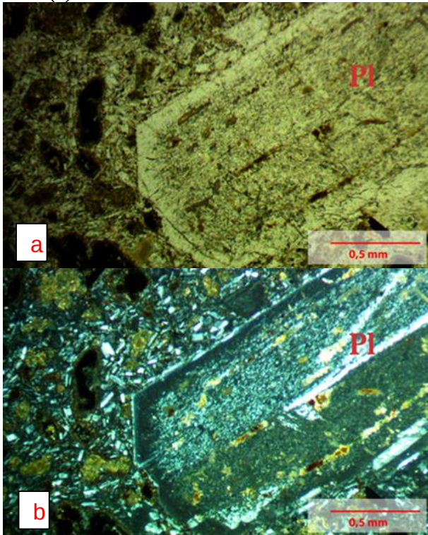
Şekil 12. Hacıilyas güneybatısından alınan yan kayaç örneklerindeki özşekilli plajiyoklaz minerallerindeki killeşme ve karbonatlaşma tek nikol (a), çift nikol (b).
