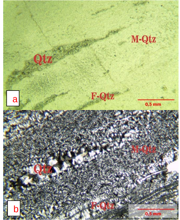
Şekil 13. YK-13 nolu kalsedon örneklerindeki kuvars (Qtz), mikrokristalin kuvars (M-Qtz) ve lifsi/iğnemsli kuvars (F-Qtz) minerallerinin tek nikol (a) ve çift nikol (b) görüntüleri.
