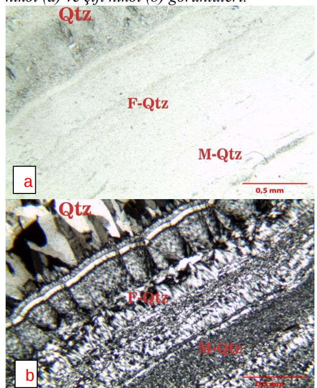
Şekil 14. YK-1 nolu kalsedon örneklerindeki kuvars (Qtz), mikrokristalin kuvars (M-Qtz) ve lifsi/iğnemsli kuvars (F-Qtz) minerallerinden oluşan laminaların ardalanması tek nikol (a) ve çift nikol (b).
